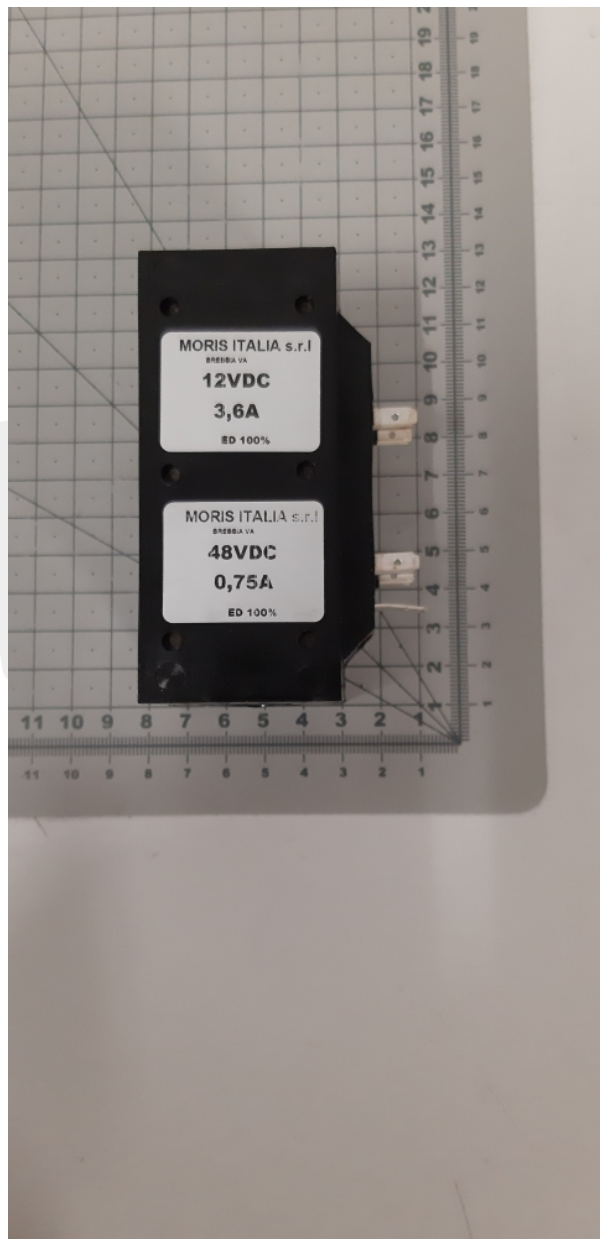
BOB/B048/12DV Cewka podwójnego napięcia 48/12 v
